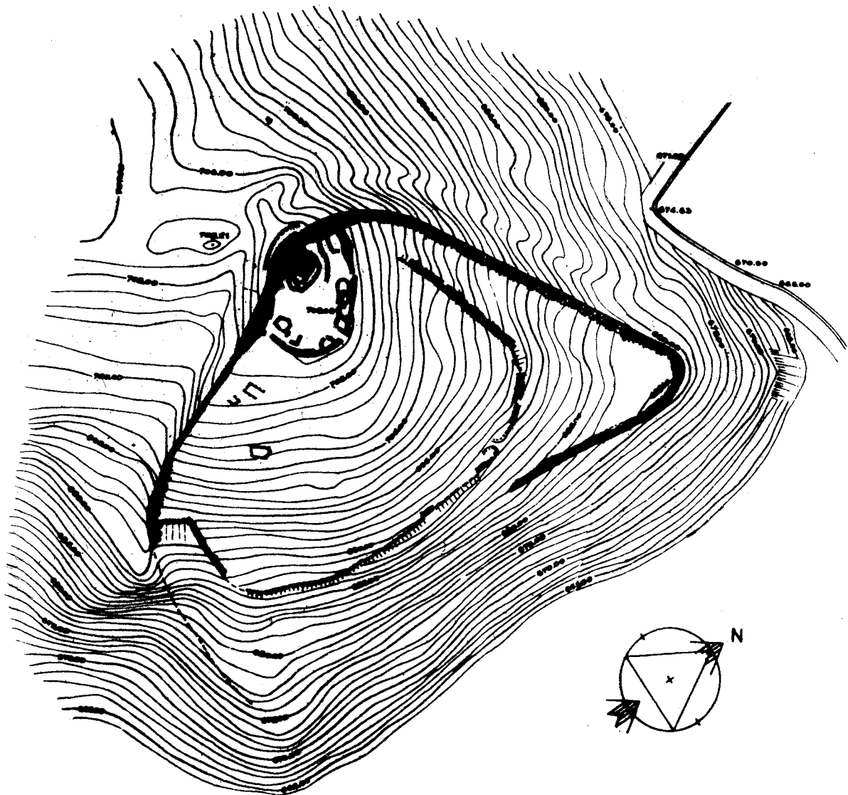
Fig. 6 — Planta topográfica do Castro de Sabrosa, segundo ERVEDOSA (1982).
