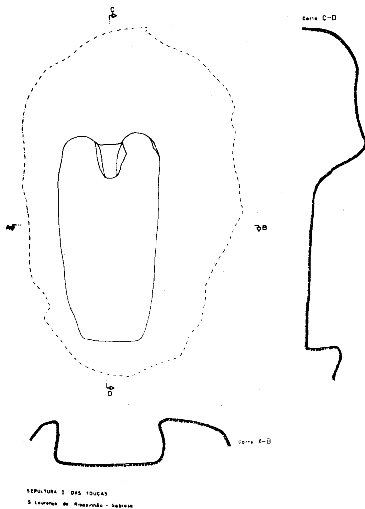
Fig. 9 — Sepultura 4 das «Touças» (S. Lourenço). Planta e secções.
