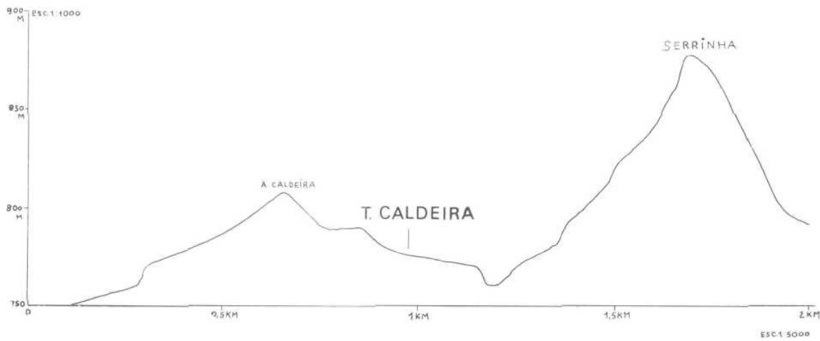
2 — Perfil OSO-ENE da Serra da Aboboreira, entre a elevação do Alto da Caldeira e a do marco geodésico da Serrinha.
