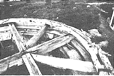
1 — Parte superior de um moinho de vento arruinado, vendo-se componentes pertencentes ao tipo de tracção por meio de grade e ao tipo de rotação por meio de sarilho interior, o que evidencia uma modificação das suas características técnicas.
